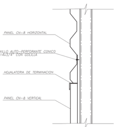
DETALLE REVESTIMIENTO HORIZONTAL Y VERTICAL
